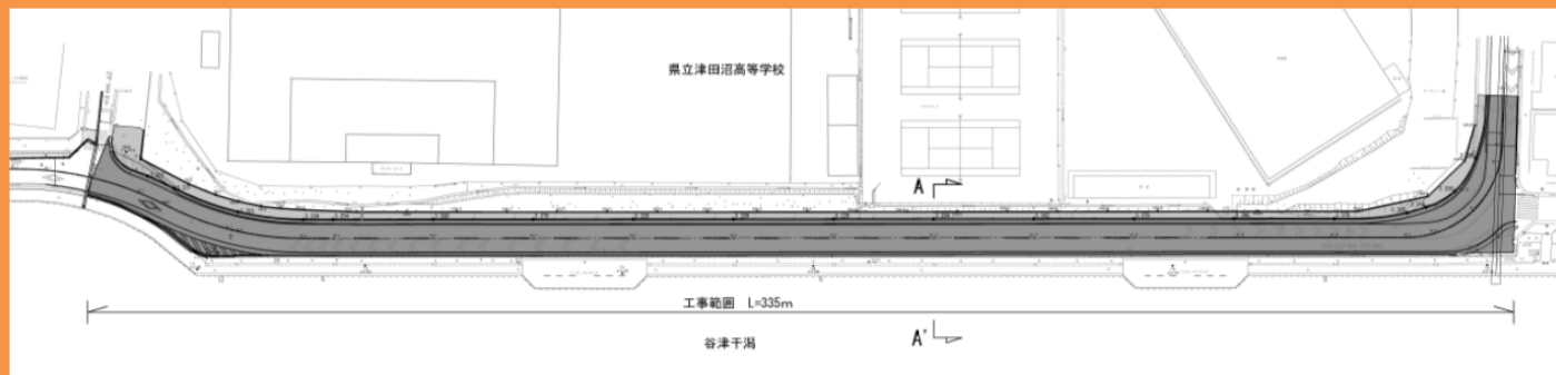
津田沼高校西側の道路拡幅 計画平面図
